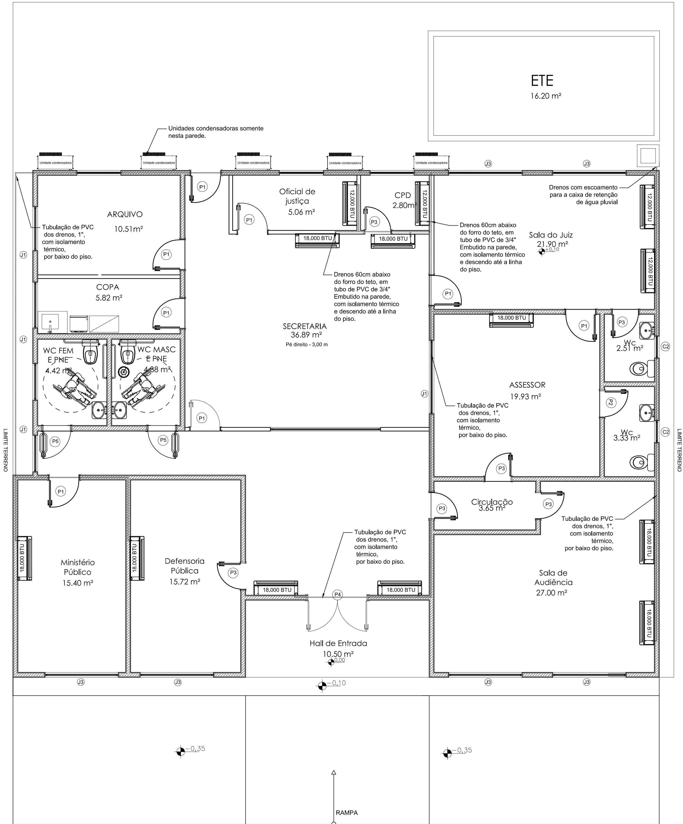
PLANTA DE AR CONDICIONADO E DRENO Esc.: 1/50
