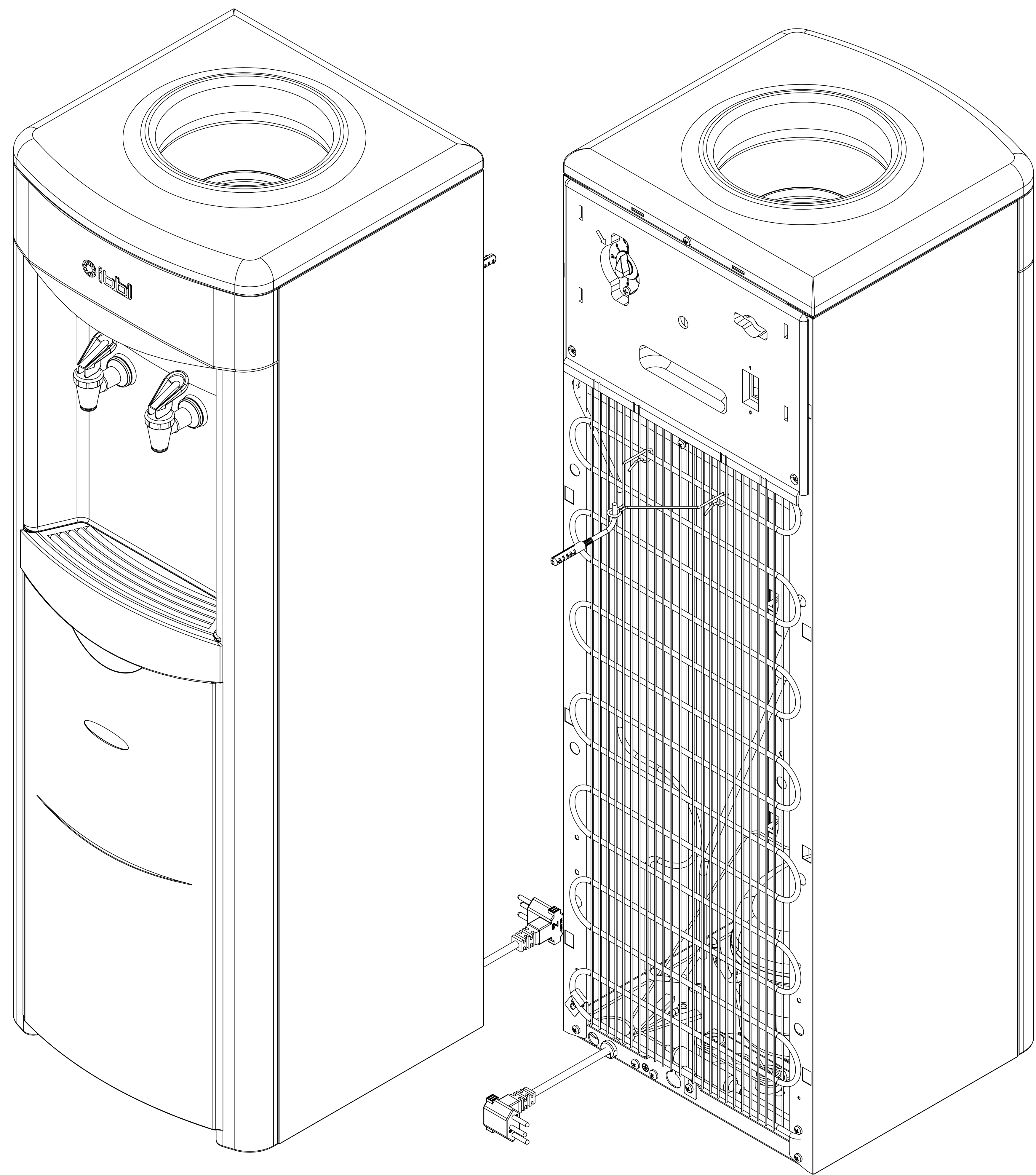
VISTA ISOMÉTRICA 1:2
