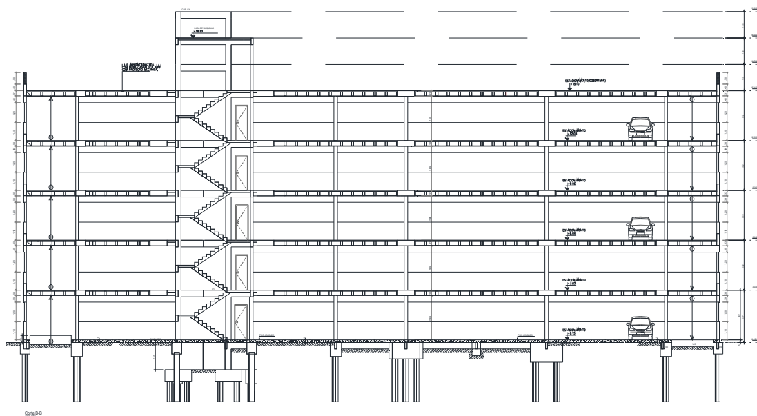
CORTE LONGITUDINAL- 01 ESCALA: 1/100
