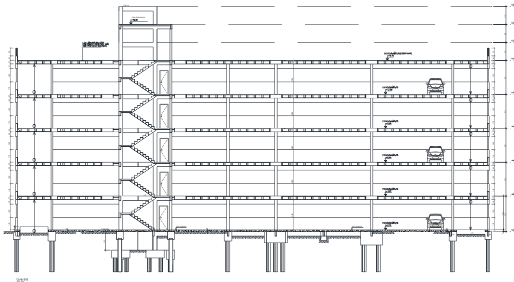
CORTE LONGITUDINAL- 01 ESCALA 1:100
