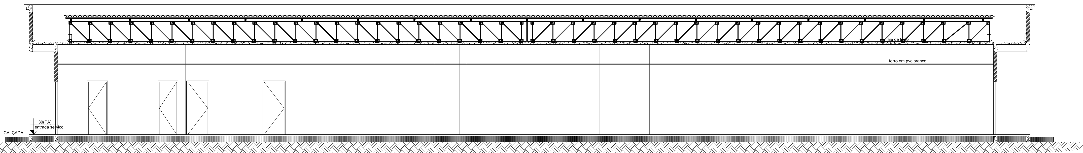
2 CORTA - ESTRUTURA METÁLICA ESC.: 1/75
