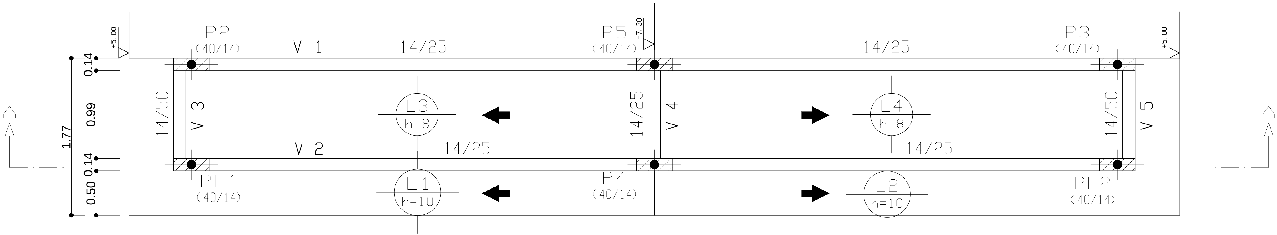
FORMA LAJE INCLINADA NÍVEL 02
