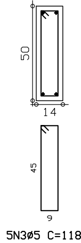
Corte A Escala 1: 20
