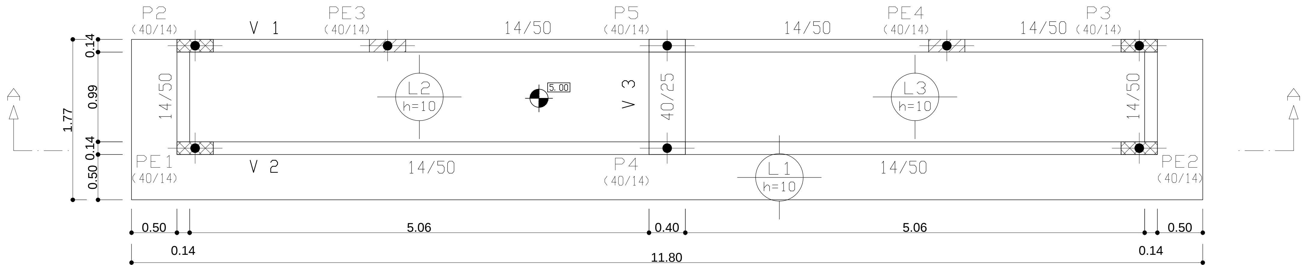
FORMA LAJE NÍVEL 01
