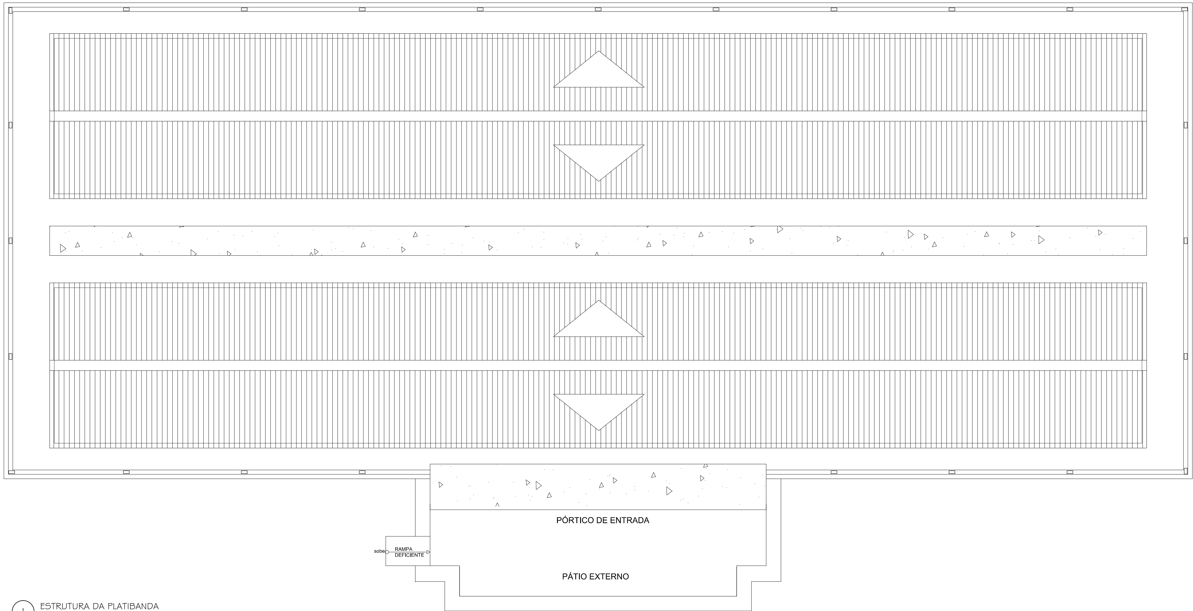
1 ESTRUTURA DA PLATIBANDA ESC.: 1/75
