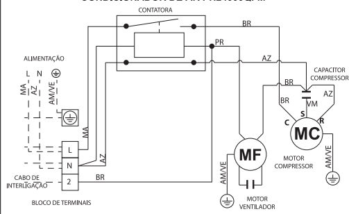
DIAGRAMA ELÉTRICO UNIDADE EXTERNA CONDICIONADOR DE AR PH24000QFM
