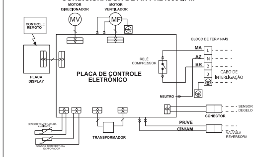
DIAGRAMA ELÉTRICO UNIDADE INTERNA CONDICIONADOR DE AR PH24000QFM
