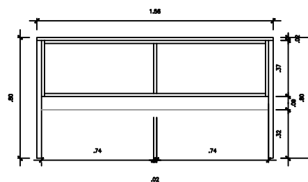
M4-Móvel para extensão da mesa Vista Posterior
