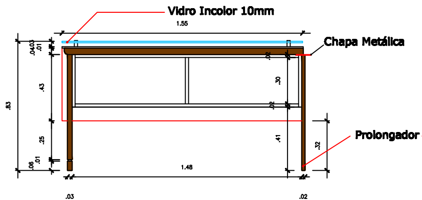
M1 - Elevação Posterior
