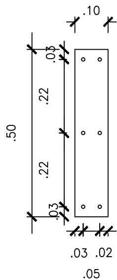
Det. em Planta Baixa do Polongador
