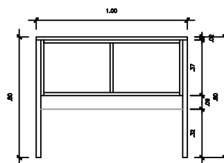
M3-Móvel para extensão da mesa Vista Posterior
