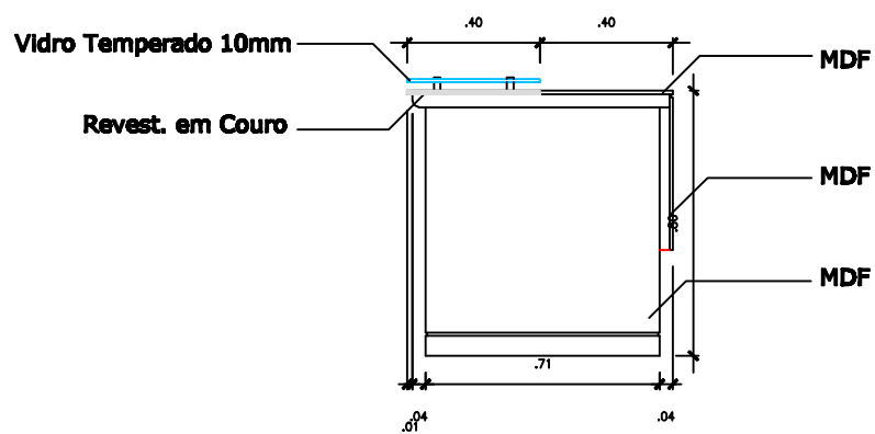
Planta 04
