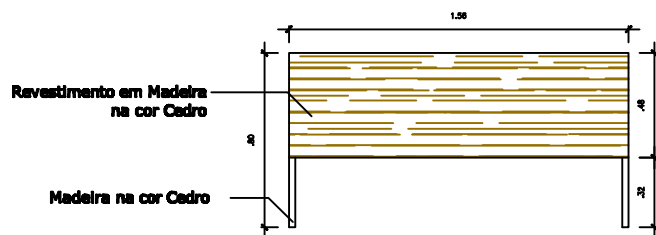
M4-Móvel para extensão da mesa Vista Frontal
