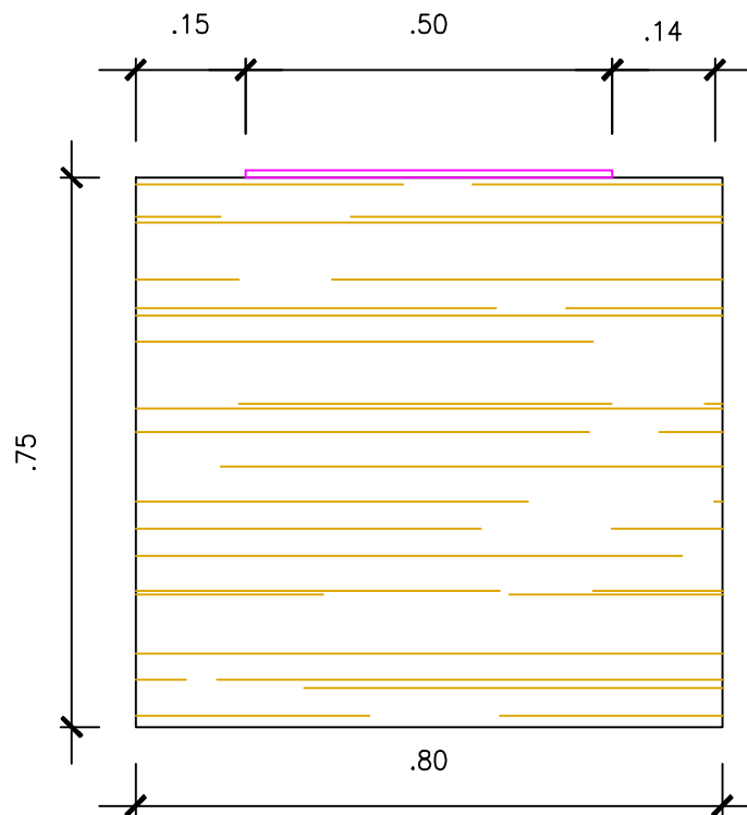
Det. em Vista Lateral do Polongador
