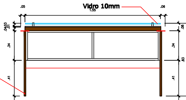
M2 - Elevação Posterior
