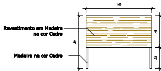
M3-Móvel para extensão da mesa Vista Frontal
