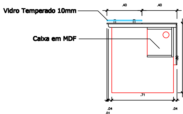
Corte 1
