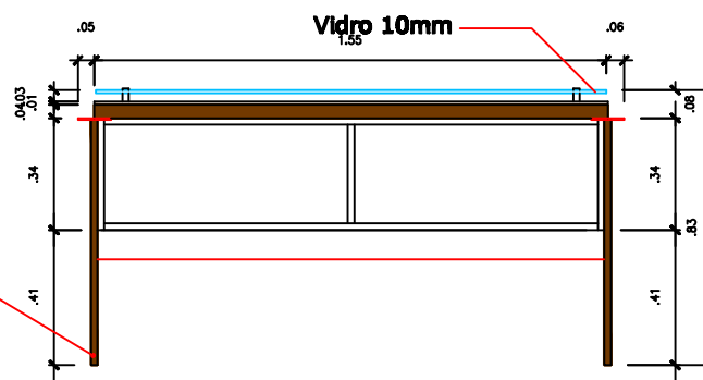
M2 - Elevação Posterior
