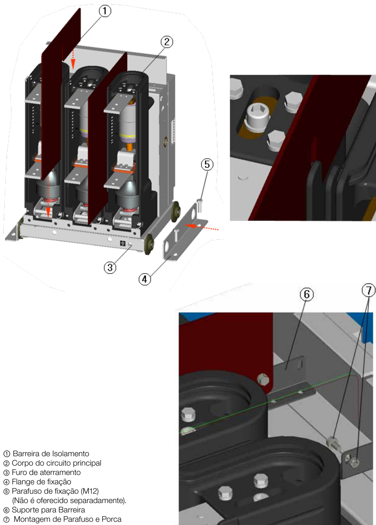
Figura 1 - Instalação do disjuntor tipo fixo.
