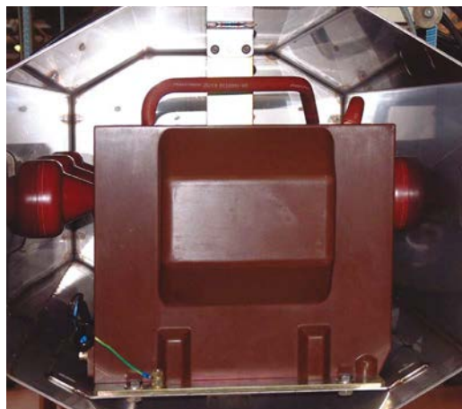
› VCS-36 Transformador de tensão tipo suporte com alimentação em interruptor aéreo de média tensão.
