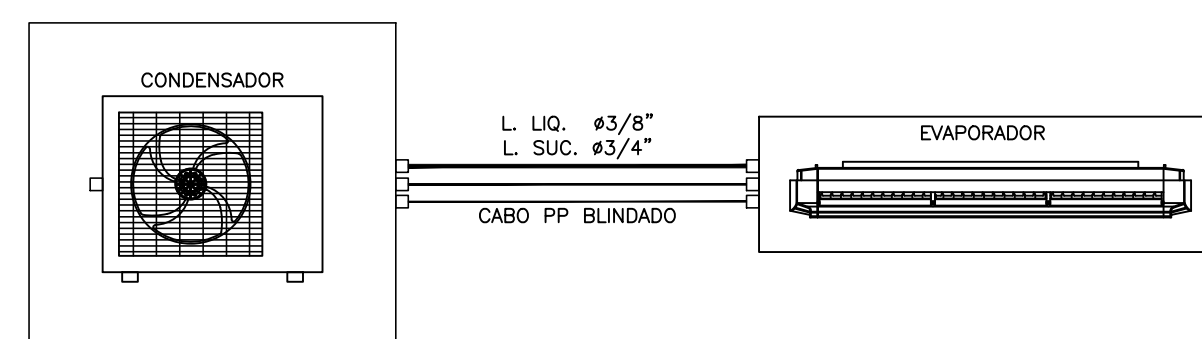
DET. 08 – LIGAÇÃO DA TUBULAÇÃO FRIGORIFICA SPLIT 36.000 BTU/h
