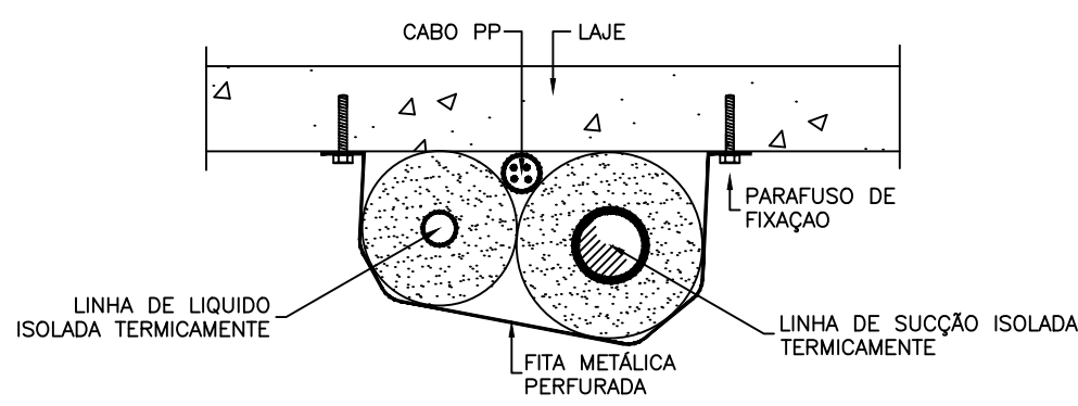
DET. 02 – INTERCONEXÃO ENTRE UNIDADES SEM ESCALA
