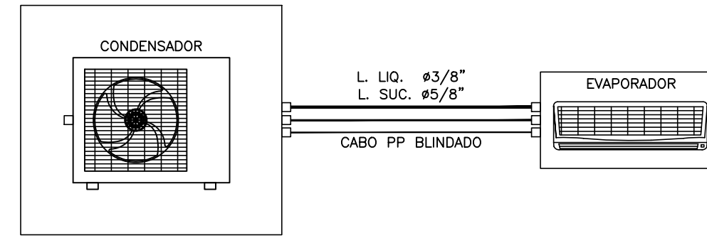
DET. 07 – LIGAÇÃO DA TUBULAÇÃO FRIGORIFICA SPLIT 24.000 BTU/h
