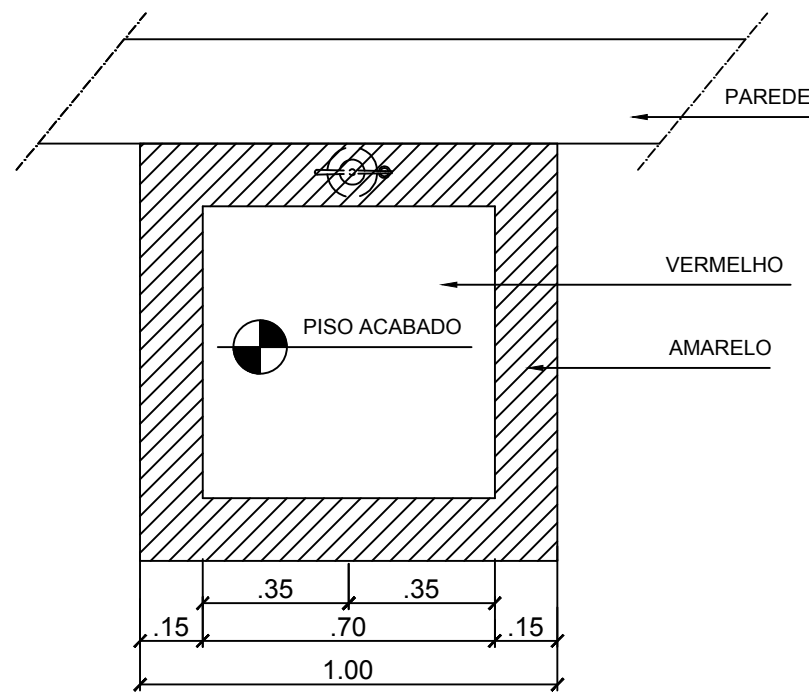
DETALHE DE MARCAÇÃO DE PISO SESCALA
