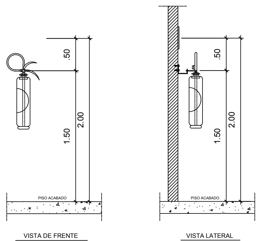
DETALHE DE MONTAGEM DOS EXTINTORES SESCALA
