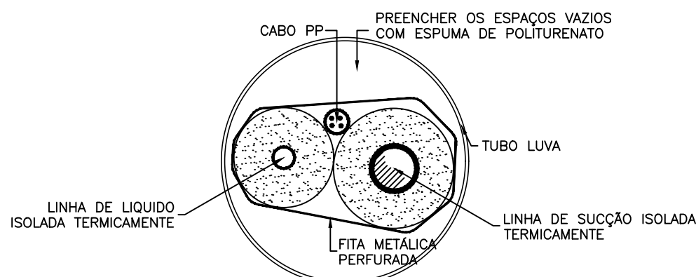
DET. 03 – MONTAGEM TUBULAÇÃO FRIGORIGENA NO TUBO LUVA SEM ESCALA
