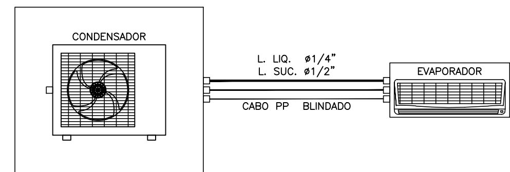
DET. 05 – LIGAÇÃO DA TUBULAÇÃO FRIGORIFICA SPLIT 12.000 BTU/h
