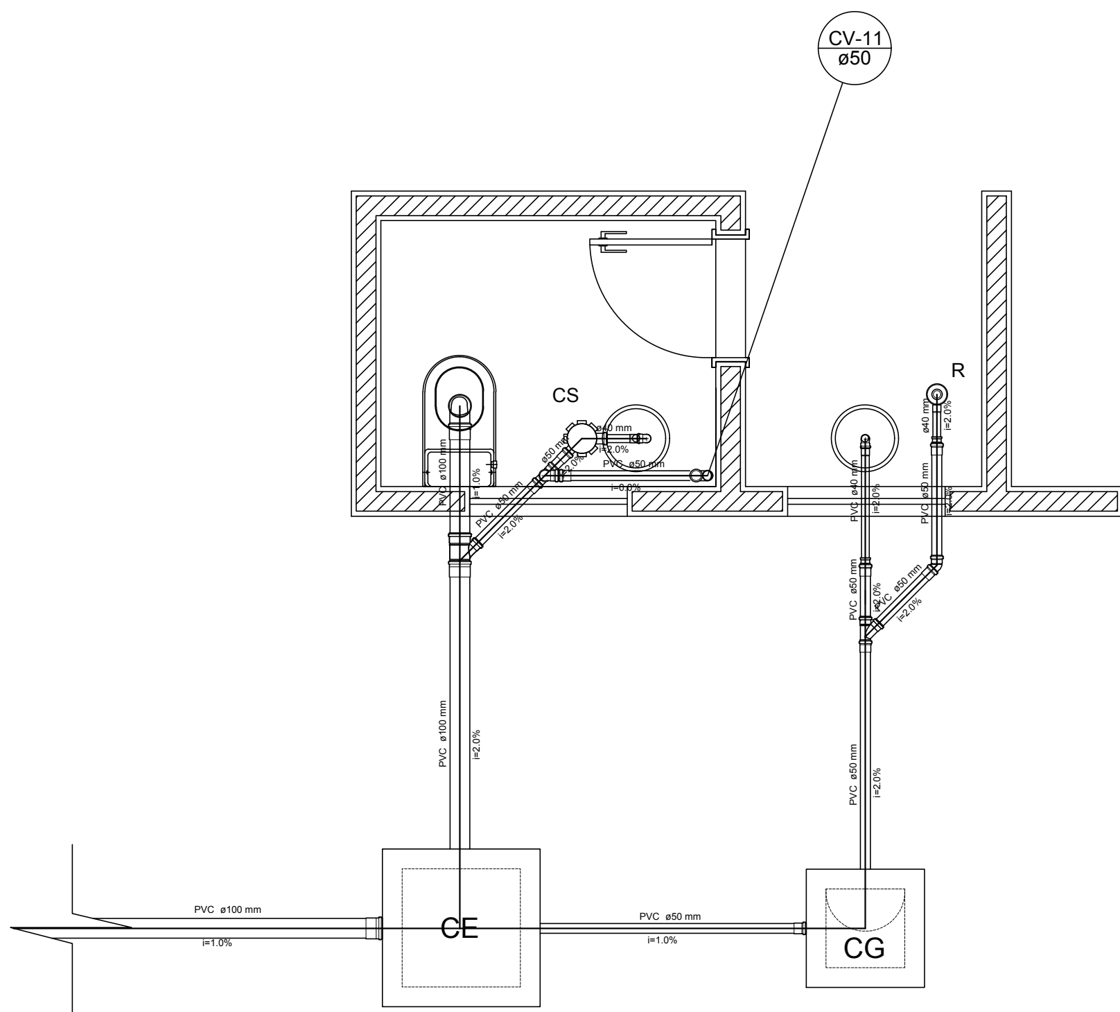
DETALHE S3 ESC.: 1/25
