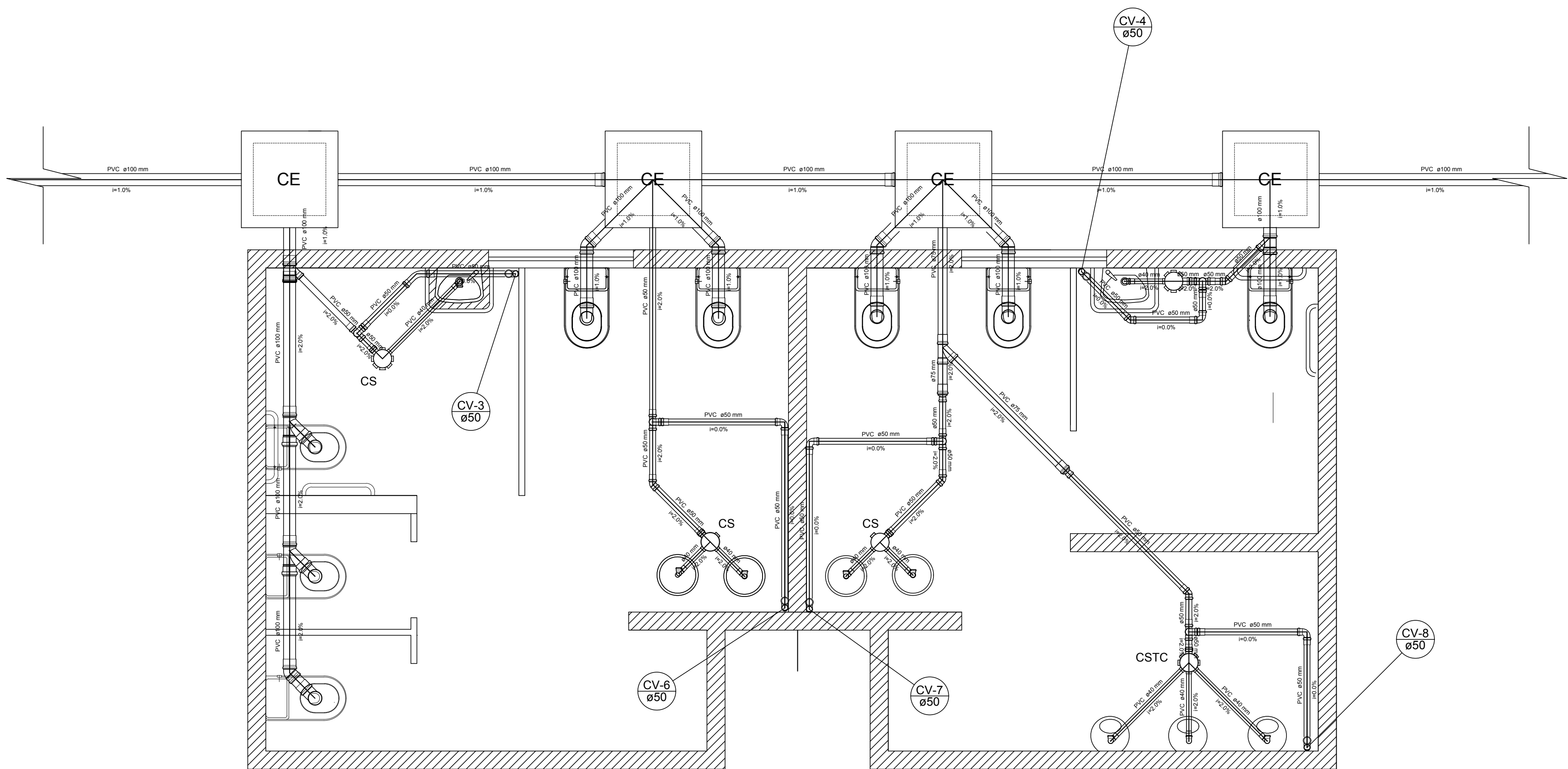
DETALHE S2 ESC.: 1/25
