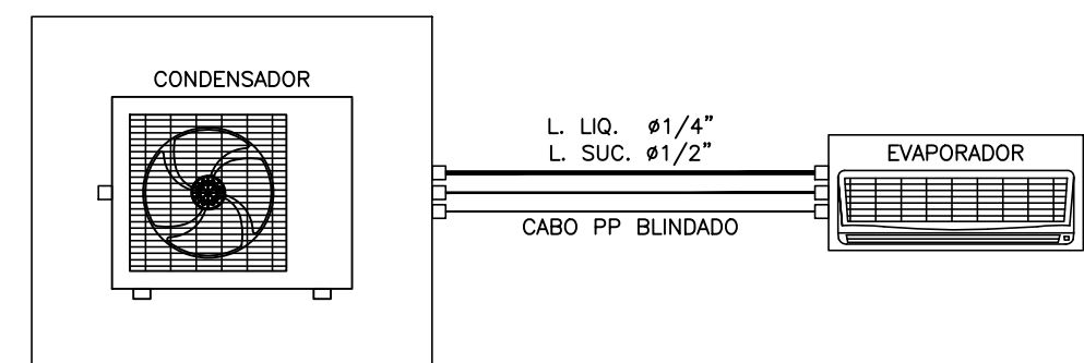
DET. 06 – LIGAÇÃO DA TUBULAÇÃO FRIGORIFICA SPLIT 18.000 BTU/h
