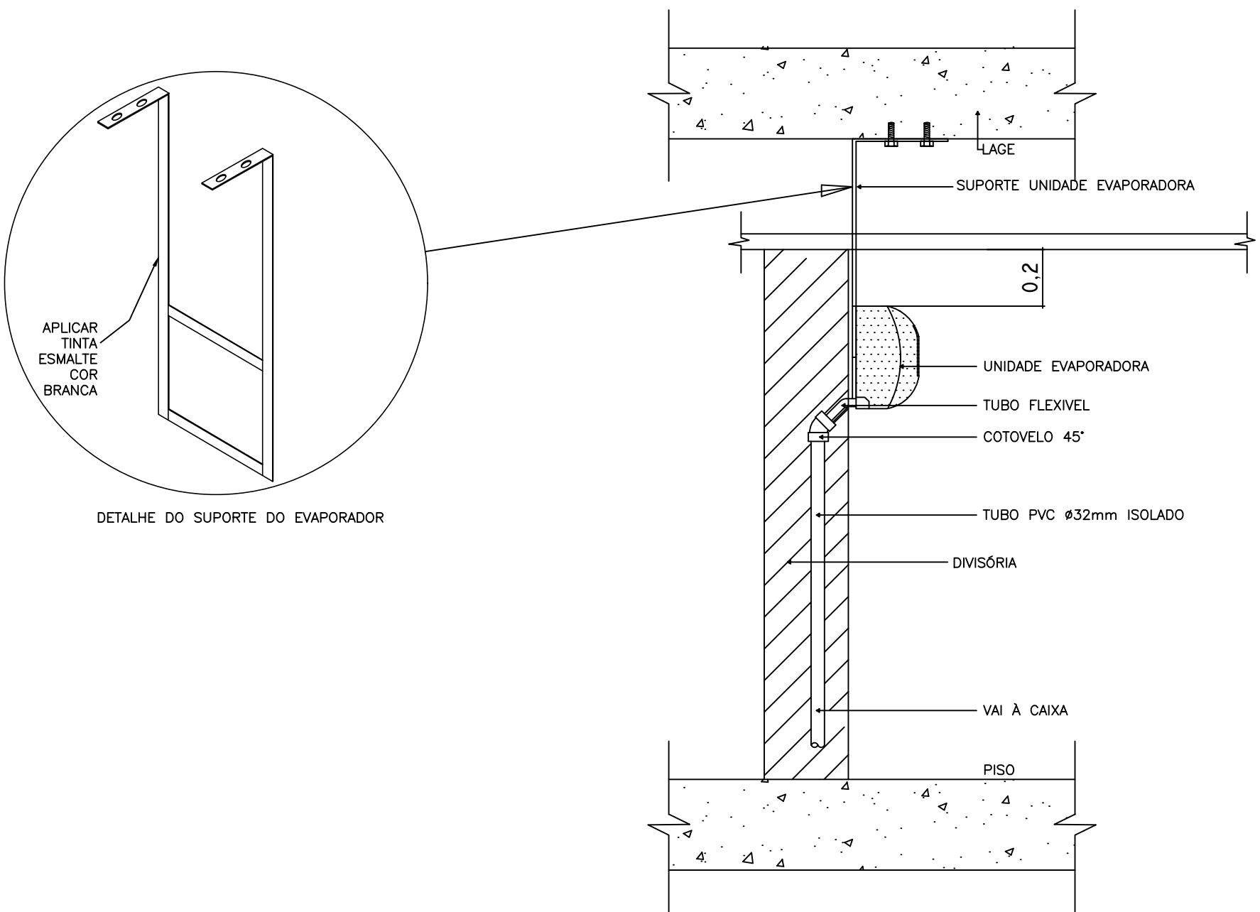
DET. 01 – INSTALAÇÃO DO DRENO SPLIT DE PAREDE ATÉ 24.000 BTU/h SEM ESCALA
