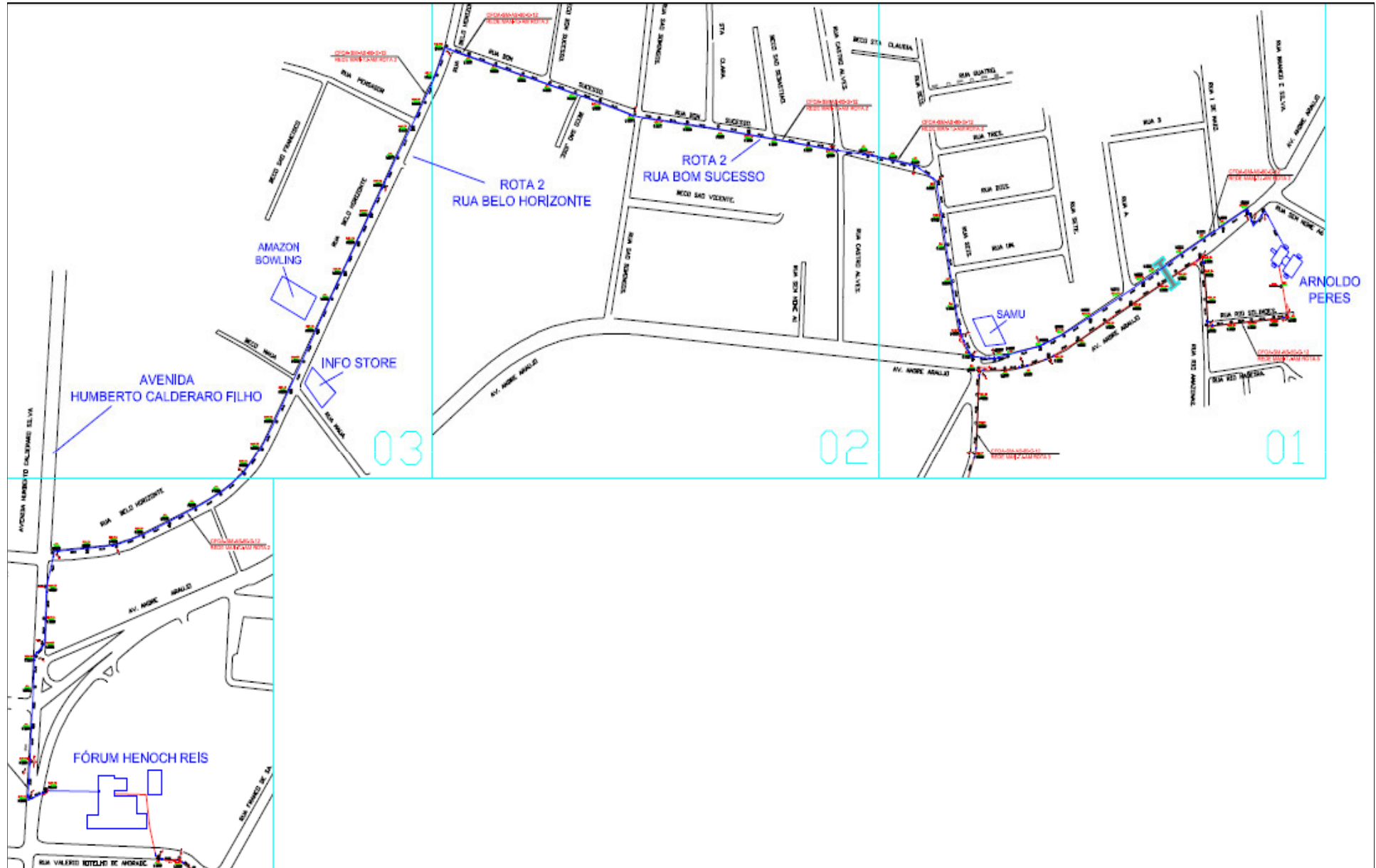
Rota 2 – Rua Belo Horizonte Comprimento da fibra : 2.343m
