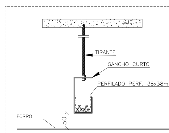
DET. 3 - VISTA FRONTAL FIXAÇÃO PERFILADOS SEM ESCALA
