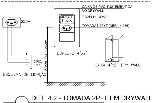
DET. 4.2 - TOMADA 2P+T EM DRYWALL SEM ESCALA
