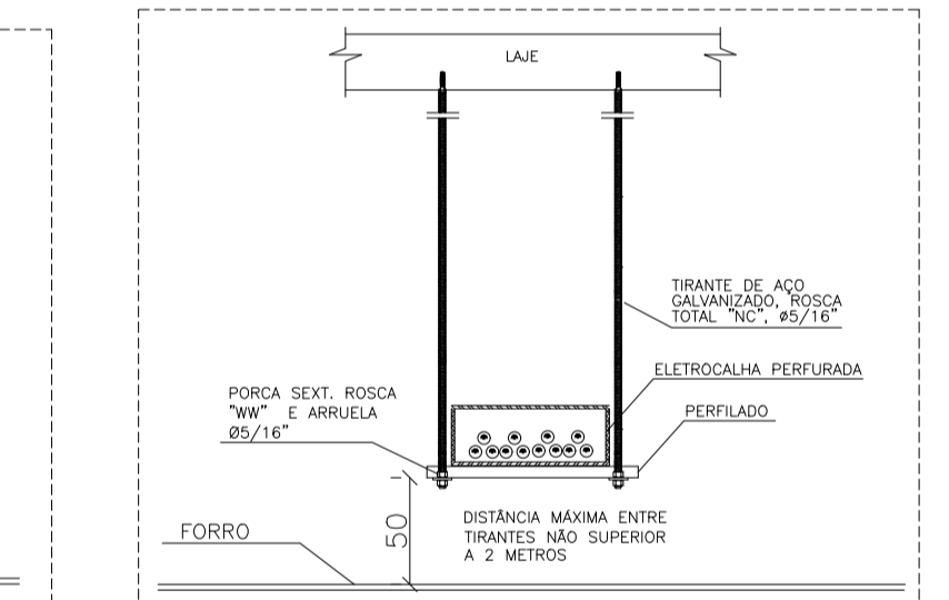
DET. 3.1 - VISTA FRONTAL FIXAÇÃO E SUPORTES P/ ELETROCALHA SEM ESCALA
