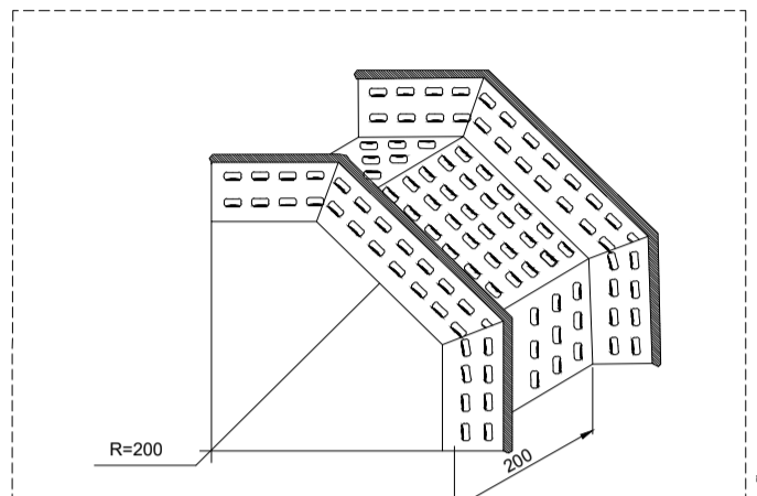
DET. 1.1 - CURVA VERTICAL EXTERNA 90° SEM ESCALA
