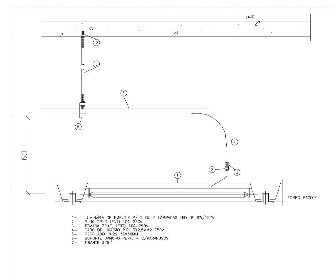
DET. 6 - LUMINÁRIA DE EMBUTIR SEM ESCALA
