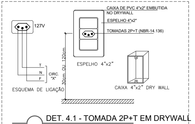
DET. 4.1 - TOMADA 2P+T EM DRYWALL SEM ESCALA
