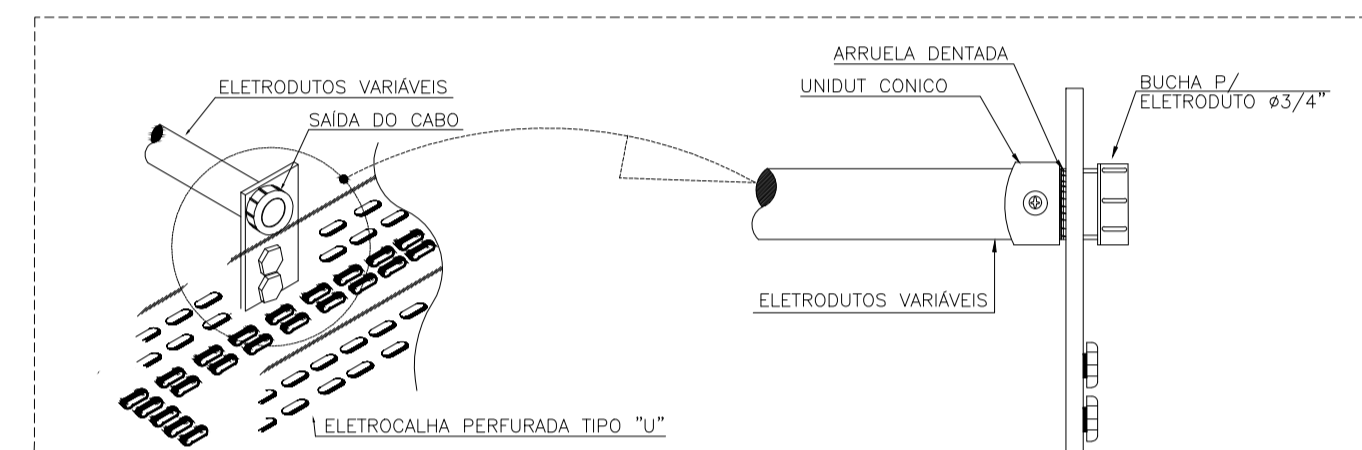
DET. 2 - ELETRODUTO ACOPLADO EM ELETROCALHA SEM ESCALA
