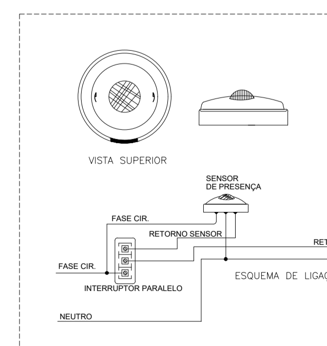
DET. 8 - ESQUEMA LIGAÇÃO SENSOR DE PRESENÇA COM INTERRUPTOR PARALELO SEM ESCALA
