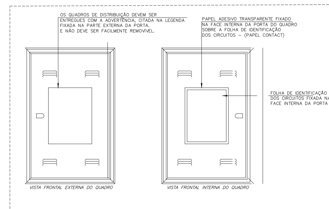
DET. 5 - ILUSTRATIVO DA VISTA FRONTAL INT./EXT. DO QUADRO DISTRIBUIÇÃO SEM ESCALA
