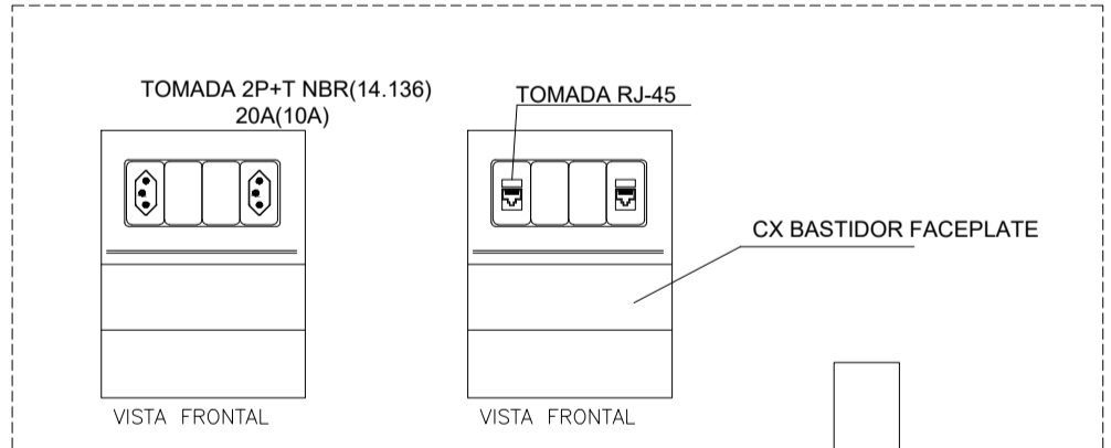
DET. 4 - DETALHE DE TOMADA 2P+T PROXIMO A TOMADA RJ-45 NA PAREDE SEM ESCALA
