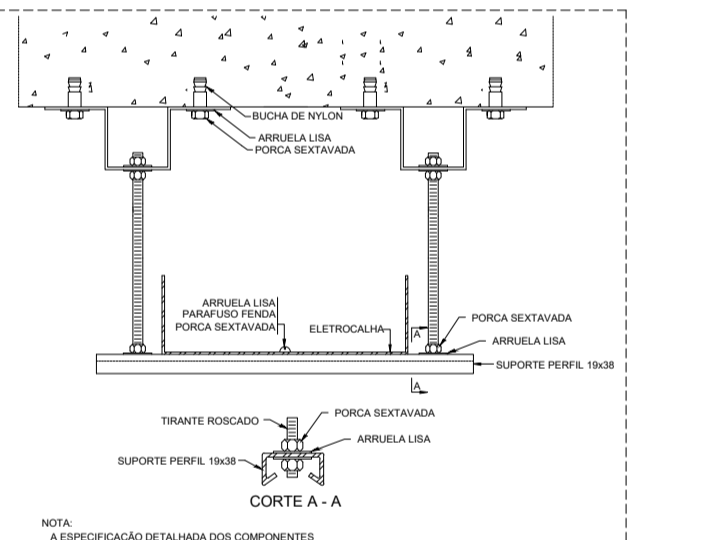
DET. 3.2 - VISTA FRONTAL FIXAÇÃO E SUPORTES P/ ELETROCALHA SEM ESCALA
