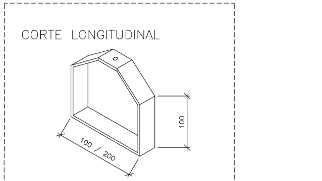
DET. 1.2 - CURVA VERTICAL EXTERNA 90° SEM ESCALA
