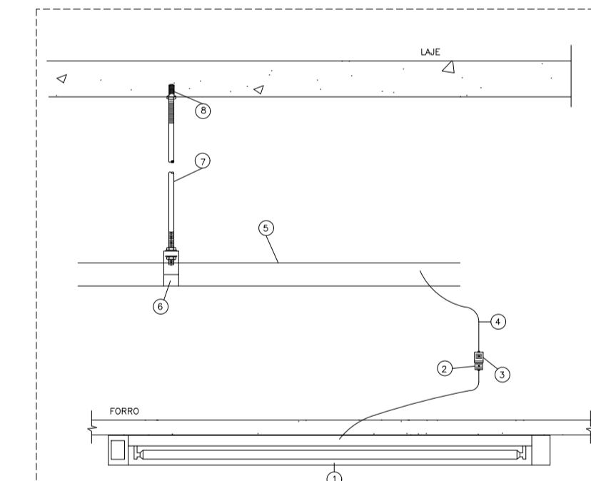
DET. 7 - LUMINÁRIA DE SOBREPOR SEM ESCALA
