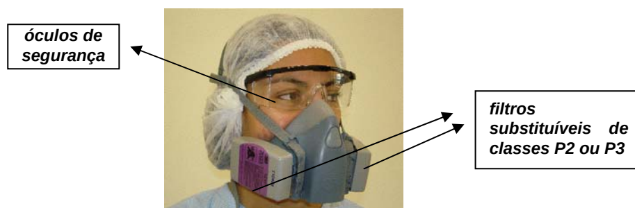
Figura 11: EPR purificador de ar com peça semifacial e filtros substituíveis de classes P2 ou P3 aos pares (Obs: os óculos de segurança não fazem parte do EPR)
