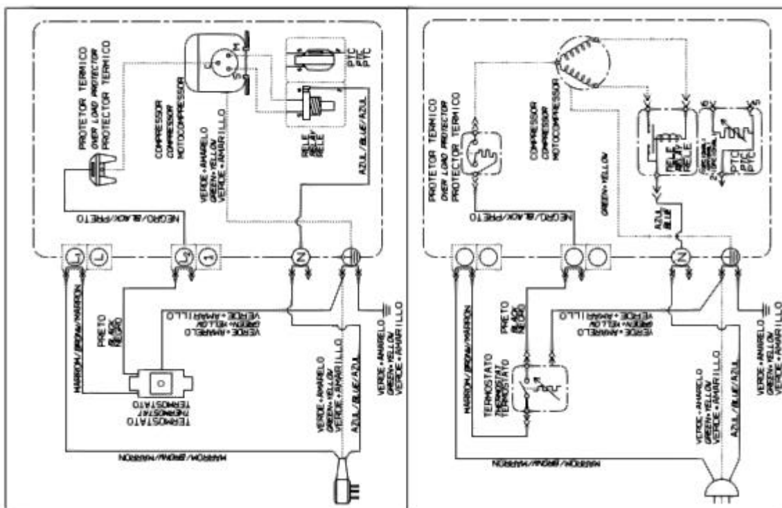
Diagrama Elétrico
