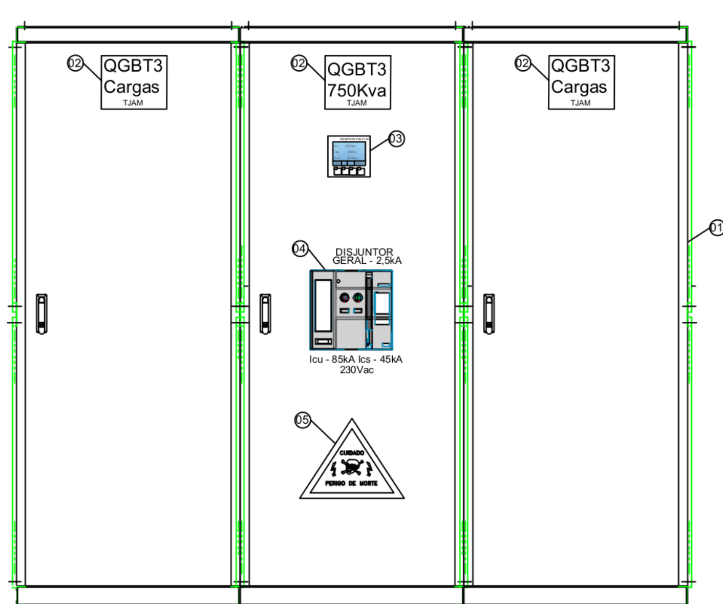
VISTA FRONTAL DO QUADRO QGBT 3 - 80 CIRCUITOS
