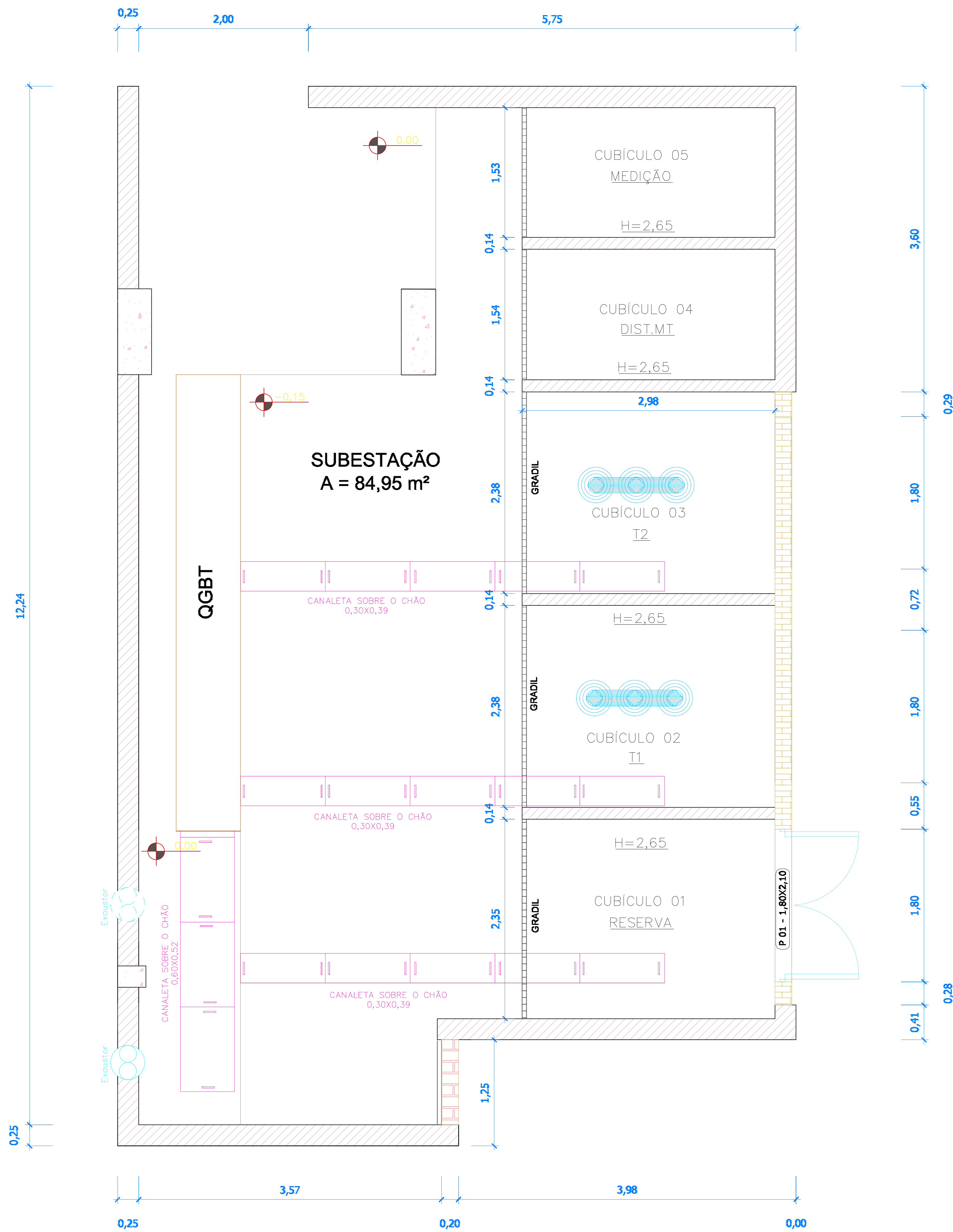
PLANTA BAIXA – SUBSOLO ESCALA: 1:75
