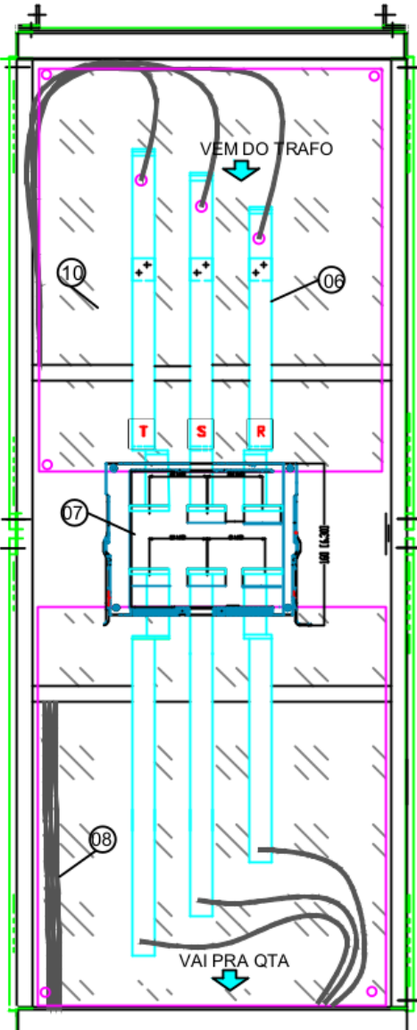
VISTA TRASEIRA INTERNA DO QUADRO QGBT 2 - GERAL
