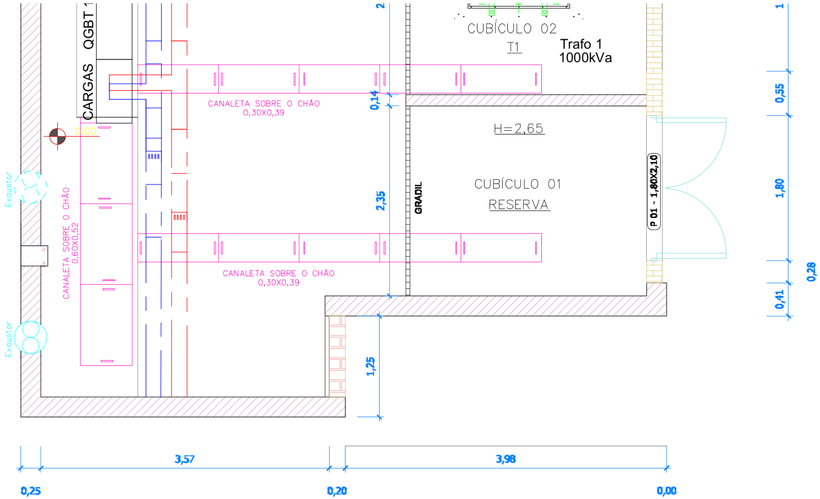
PLANTA BAIXA – SUBSOLO ESCALA: 1:75
