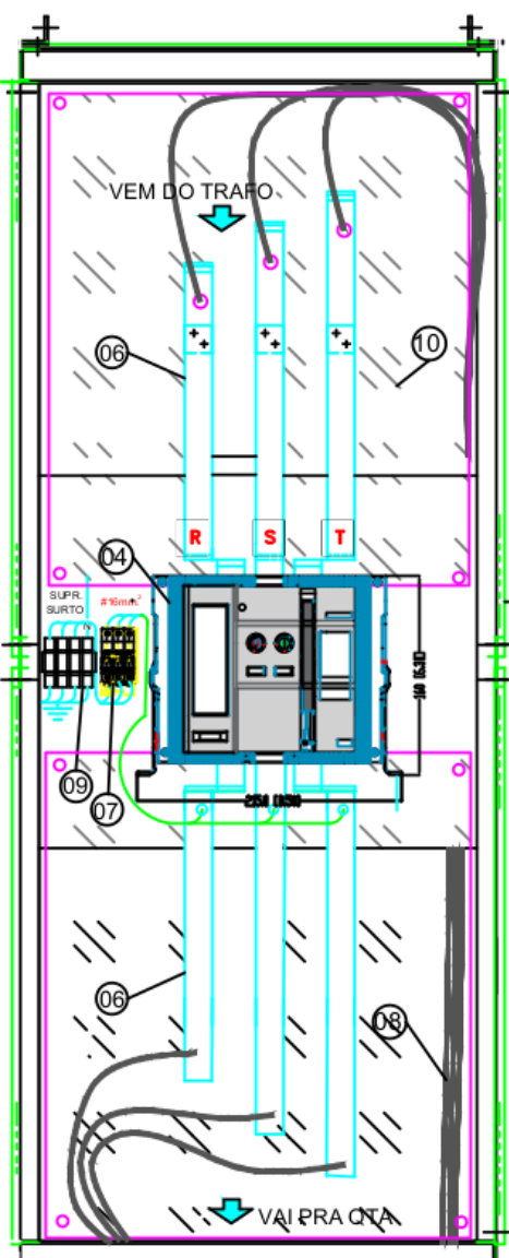
VISTA FRONTAL INTERNA DO QUADRO QGBT 2 - GERAL
