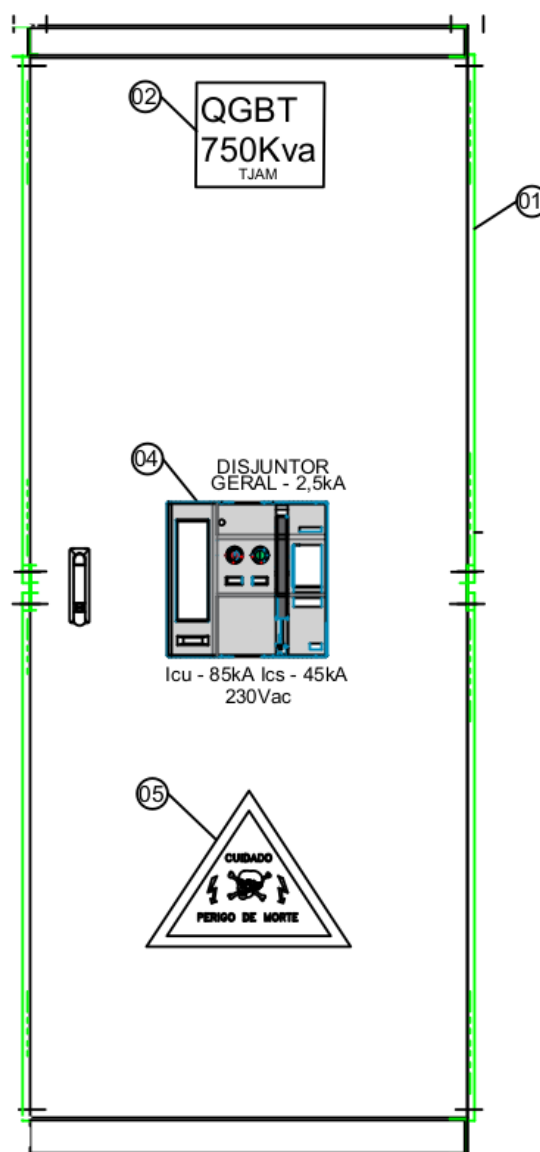
VISTA FRONTAL DO QUADRO QGBT 2 - GERAL
