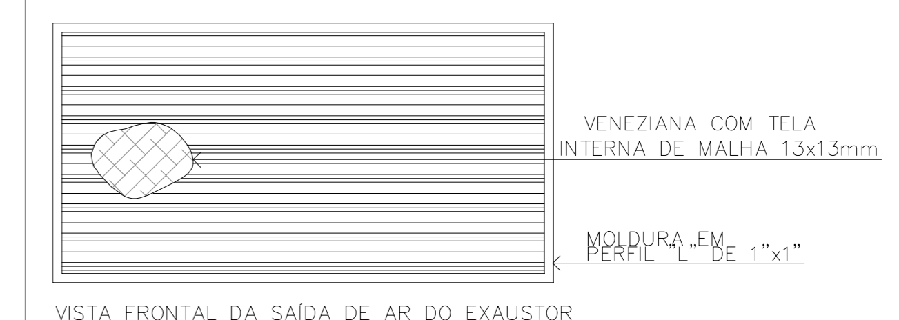
DETALHE 04 - MÓDULO DE VENTILAÇÃO S/ ESCALA
